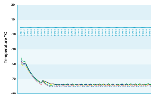
Exemplo de um Mapeamento Multitemperatura com 9 sondas dentro de um freezer vertical ULT
